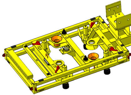
Рама выравнивающая
