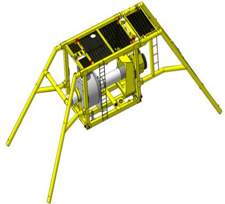
Рама защитная с трубной обвязкой (Оснащена системой мягкой посадки)
