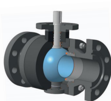
КРАНЫ ШАРОВЫЕ РАЗБОРНЫЕ ИЗ ТРЕХ ЧАСТЕЙ DN от 10 до 1400 мм, PN от 10 до 400 кгс/см 2 .
