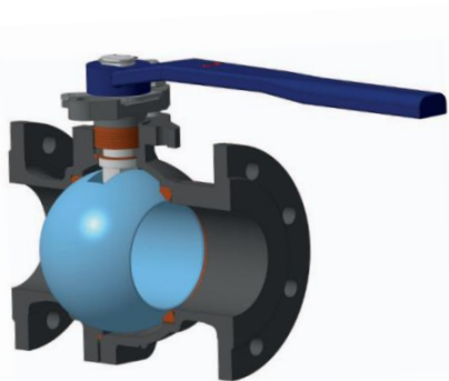
КРАНЫ ШАРОВЫЕ РАЗБОРНЫЕ ИЗ ДВУХ ЧАСТЕЙ (кованые/литые) DN от 10 до 400 мм, PN от 10 до 40 кгс/см 2 .
