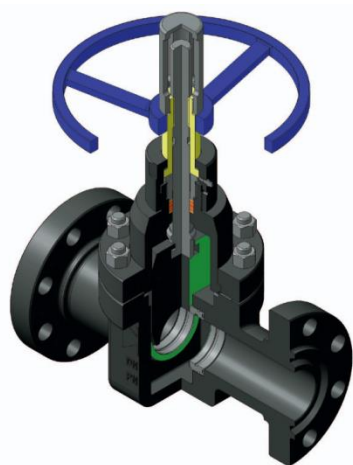
ЗАДВИЖКИ ШИБЕРНЫЕ DN от 50 до 1400 мм , PN от 10 до 1400 кгс/см 2 .
