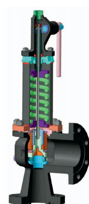
КЛАПАНА ПРЕДОХРАНИТЕЛЬНЫЕ СТАЛЬНЫЕ ПРУЖИННЫЕ с сильфоном и устройством для ручного открывания
