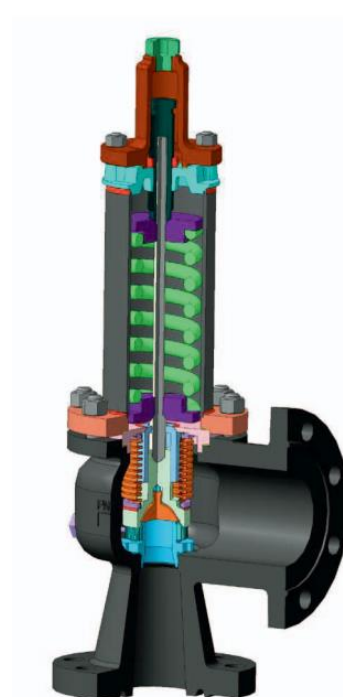
КЛАПАНА ПРЕДОХРАНИТЕЛЬНЫЕ СТАЛЬНЫЕ ПРУЖИННЫЕ с сильфоном
