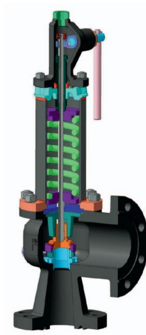
КЛАПАНА ПРЕДОХРАНИТЕЛЬНЫЕ СТАЛЬНЫЕ ПРУЖИННЫЕ с устройством ручного открывания
