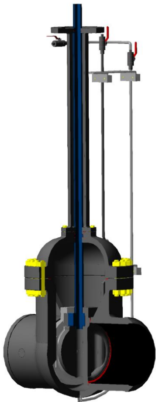
Бессальниковые задвижки DN 150-700 PN 10-250
