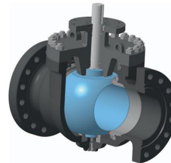
КРАНЫ ШАРОВЫЕ РАЗБОРНЫЕ С ВЕРХНЕЙ КРЫШКОЙ DN от 50 до 1200 мм, PN от 10 до 400 кгс/см 2 .
