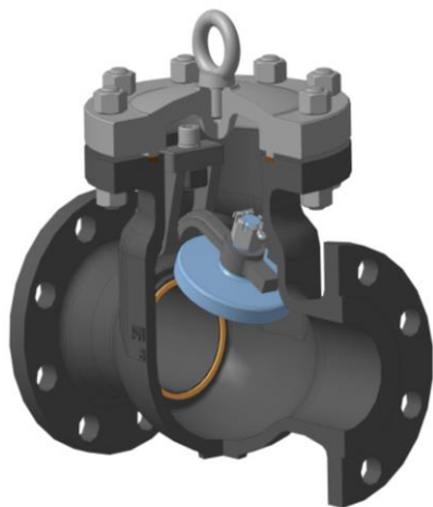
ЗАТВОРЫ ОБРАТНЫЕ (клапаны обратные поворотные) DN от 10 до 1400 мм, PN от 10 до 400 кгс/см 2 .
