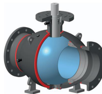
КРАНЫ ШАРОВЫЕ ЦЕЛЬНОСВАРНЫЕ ИЗ ДВУХ ЧАСТЕЙ DN от 300 до 1400 мм, PN от 10 до 125 кгс/см 2 .
