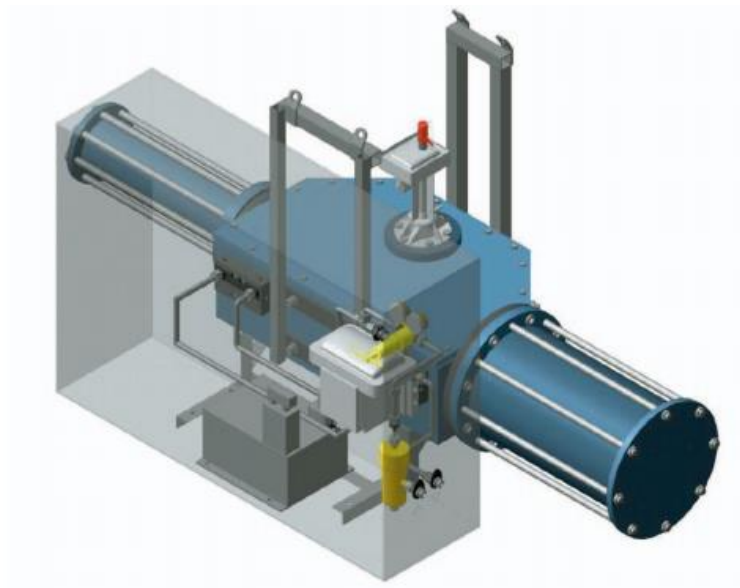
ПНЕВМОГИДРАВЛИЧЕСКИЙ ПРИВОД ДВУХСТОРОННЕГО ДЕЙСТВИЯ С КУЛИСНЫМ МЕХАНИЗМОМ И ГИДРАВЛИЧЕСКИМ ДУБЛЕРОМ
